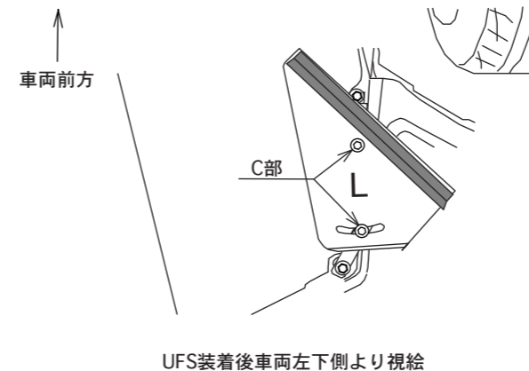
UFS装着後車両左下側より視絵
