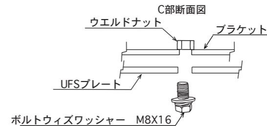
ボルトワッシャー M8X16
