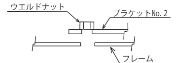
B部断面図
