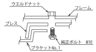
A部断面図
