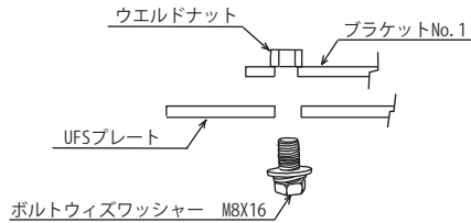
E部断面図
