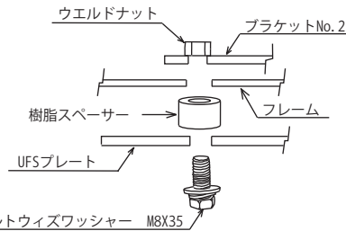
F部断面図
