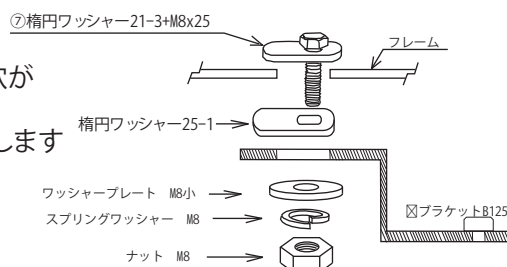
A部断面図
