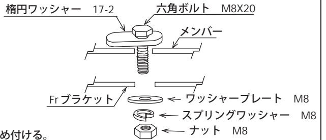
B部断面図
