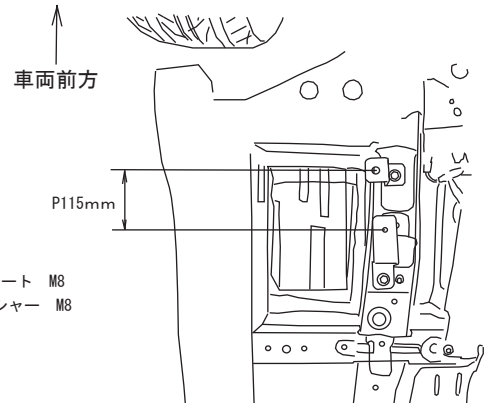
ブラケット取付後車両右下側より視絵
