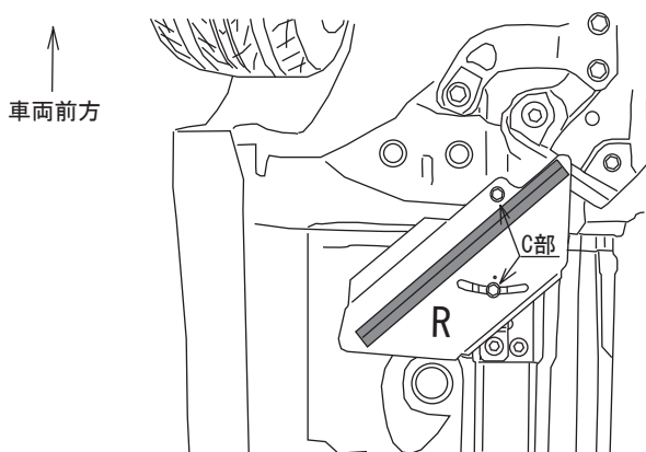
UFS装着後車両右下側より視絵
