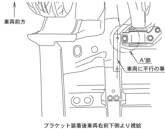
ブラケット装着後車両右前下側より視絵
