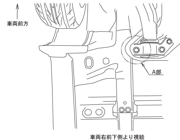
車両右前下側より視絵
