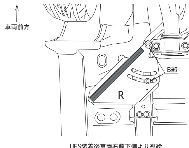
UFS装着後車両右前下側より視絵
