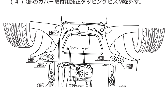
車両前方アンダーカバー真下より視絵
