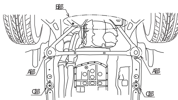
車両前方プレス真下より視絵
